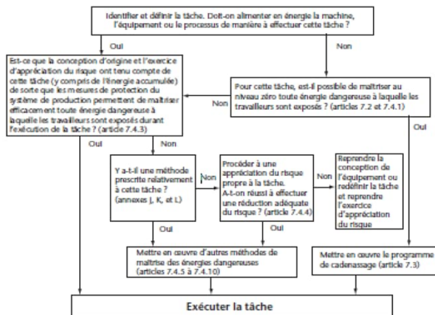
Figure 3 Logique décisionnelle relative à la sélection d'une méthode de maîtrise des énergies dangereuses (voir les articles 7.2 et 7.4.1)
